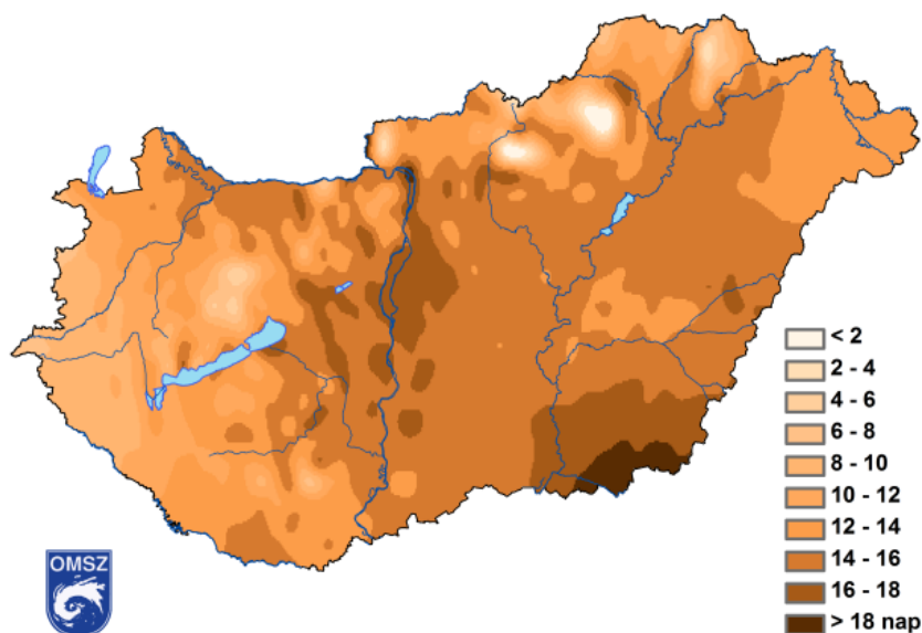
A hőhullámos napok (napi középhőmérséklet > 25^{\circ}\text{C} ) változásának területi jellemzői az 1981–2015 időszakra (Forrás: Országos Meteorológiai Szolgálat, NÉS-2)
